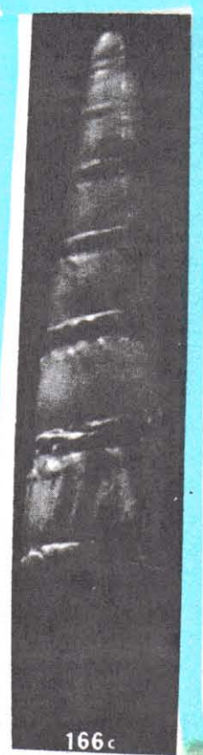
166c, Damaged holotype of T. patagonica d'Orbigny, British Museum (N.H.) No. 1854.12.5.501.; 48.8 mm.
